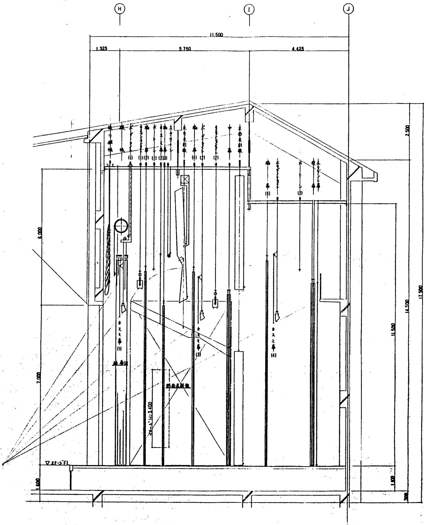
舞台平面装置断面図 1/50
